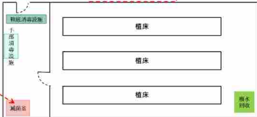
000溫室配置圖
